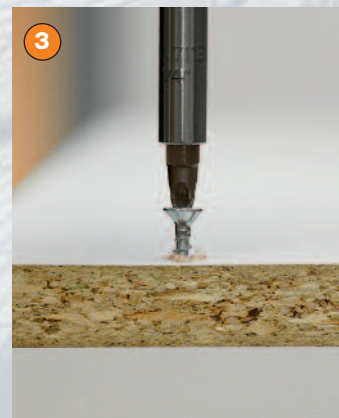
3 Dank der kleineren Gewindesteigung werden die Bauteile schon jetzt zusammengezogen
