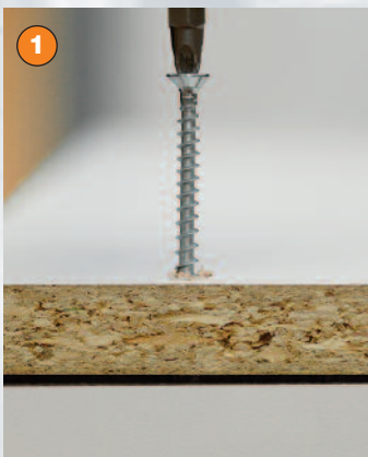
1 Der Spalt beim Verschrauben der Bauteile ist deutlich zu sehen
