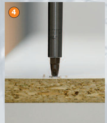
4 Versenkung des Kopfes für ein ansprechendes Verschraubbild
