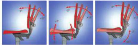
Ausführung A mit Bodengleitern
